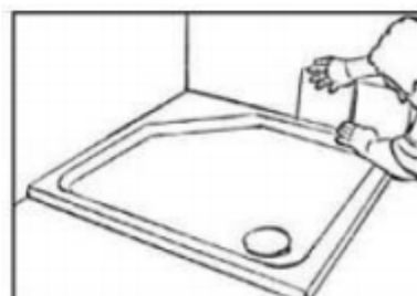
8. Przyklejenie płytek ściennych umieszczając je pomiędzy brodzikiem a ścianą
