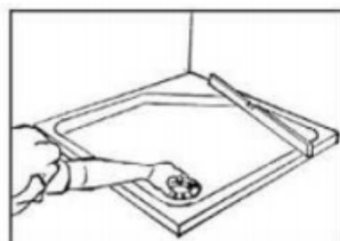
7. Wypoziomowanie brodzika, przykręcenie górnego elementu syfonu
